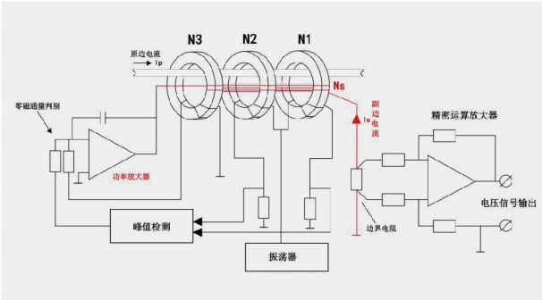
磁通门传感器的整体框图
